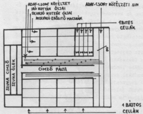
3. ÁBRA. AZ EBAM Belső FELÉPÍTÉSÉNEK VÁZLATA
